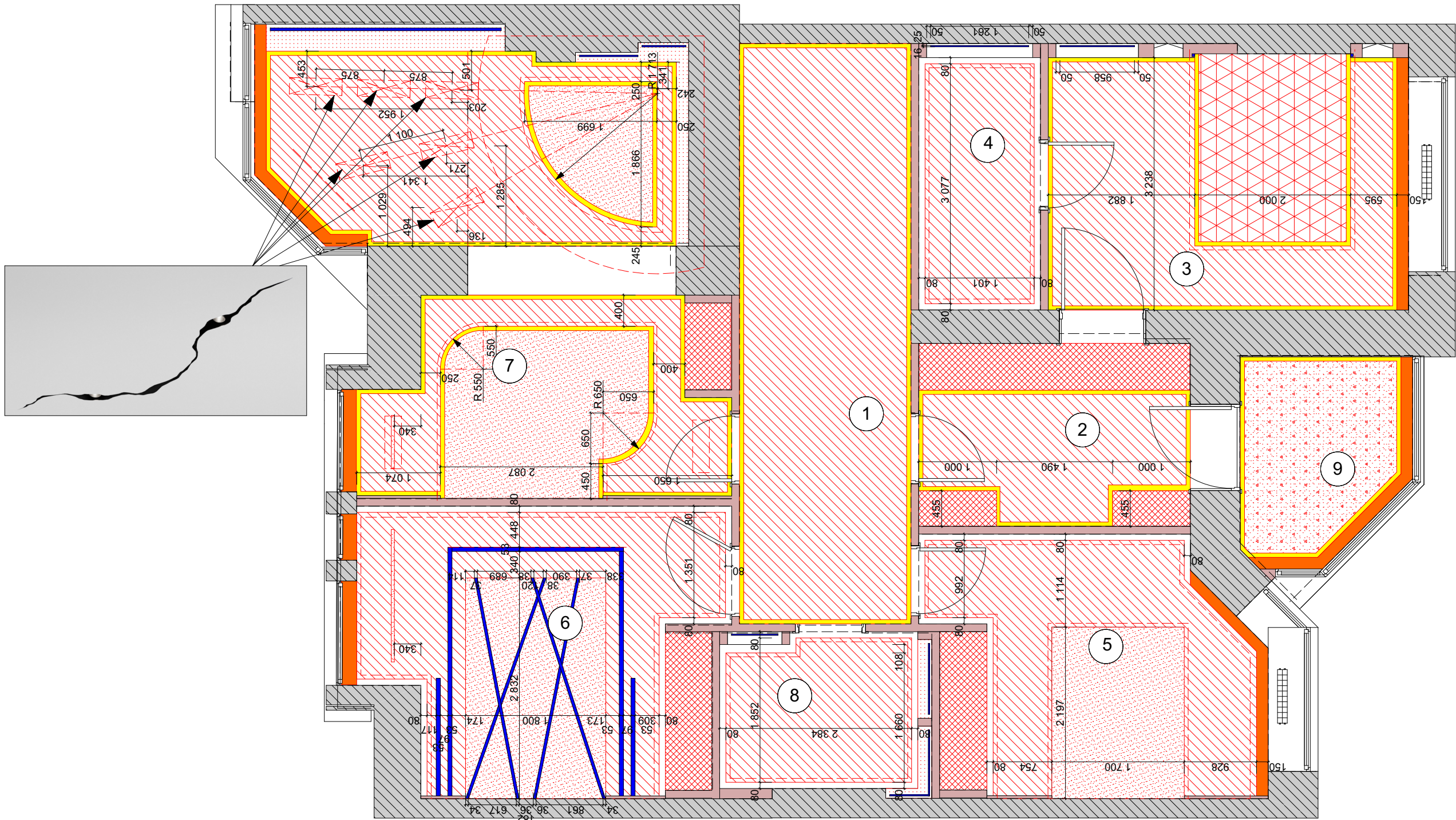
ЭКСПЛИКАЦИЯ ПОМЕЩЕНИЙ:
